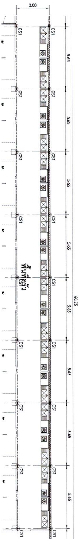
แปลนเสาเอ็นหลังคา มาตราส่วน 1 : 150
