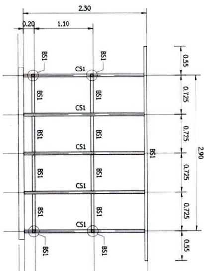
แบบโครงสร้างกลาง ขนาดหน้ากว้าง 2.30 ม. 1 : 50
