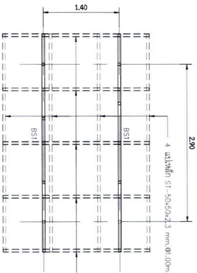
แบบโครงสร้างท่อนบน ขนาดหน้ากว้าง 1.40 ม. 1 : 50
