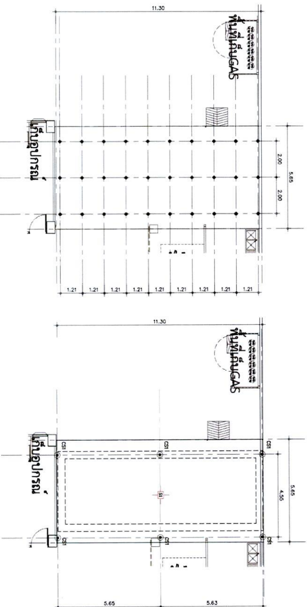
แปลนเสาเข็ม SCALE 1:100
