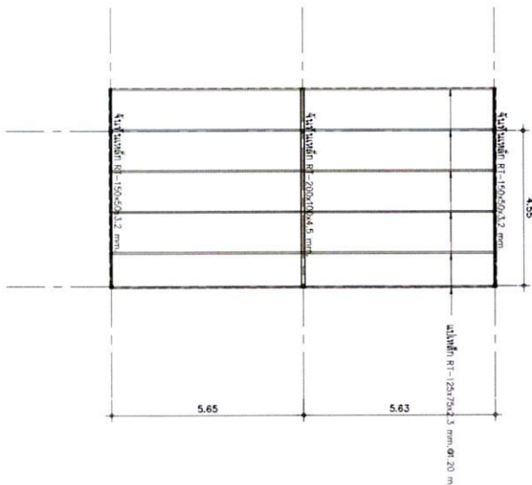
แปลนโครงสร้างพื้น SCALE 1:100
